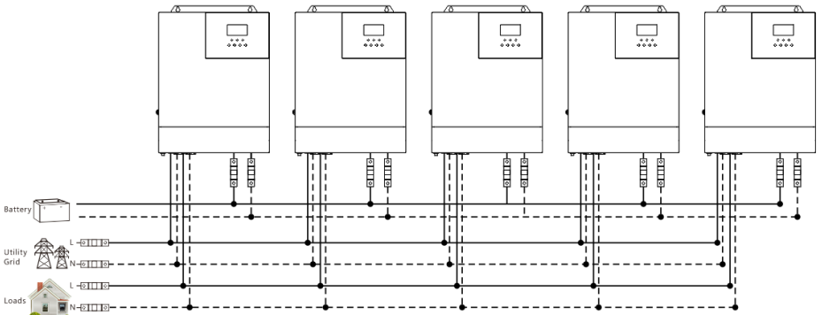
d) 系统五台逆控一体机并联：
