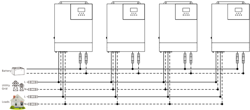
c) 系统四台逆控一体机并联：
